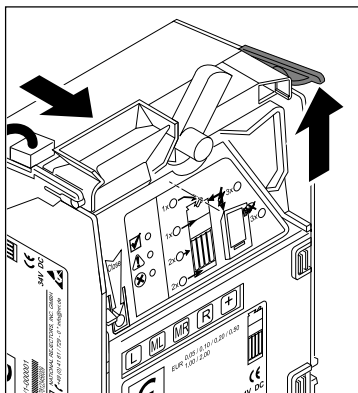
Abb. 1b: Münzprüfer ausbauen
