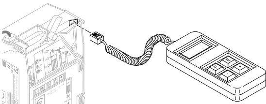
Abb. 7c: Anschluss an Einstellmodul
